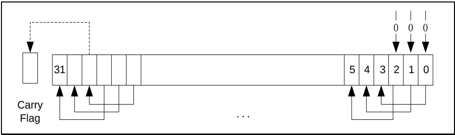
附录图 1-10LSL #3
