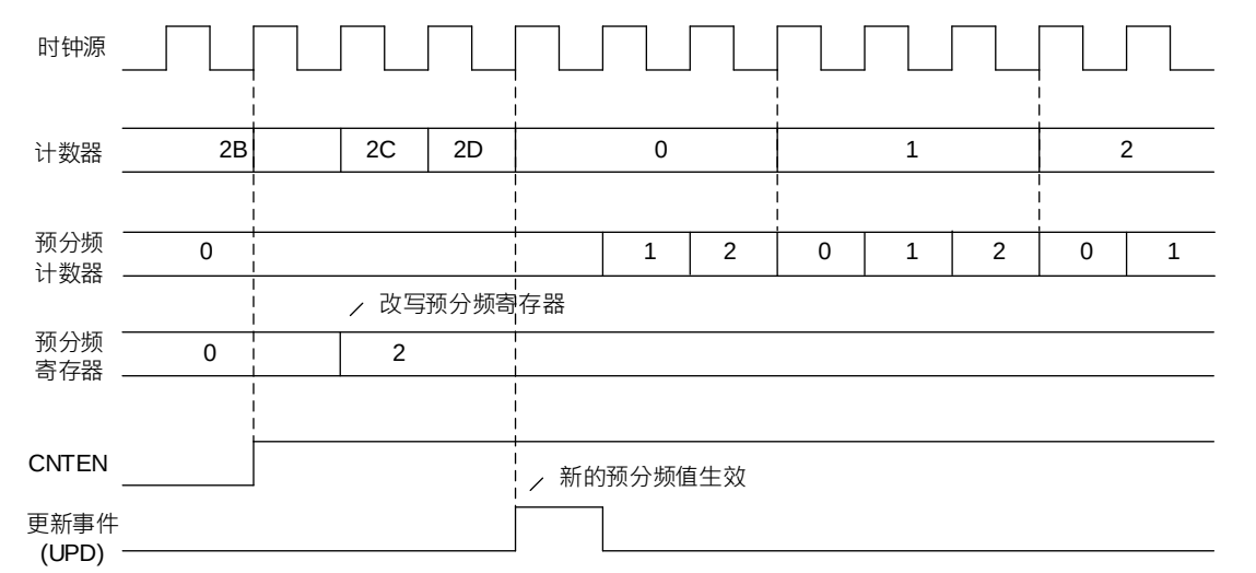
图 20-2 预分频值计数时序图
