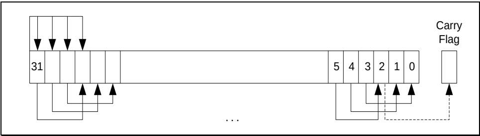
附录图 1-8ASR #3
