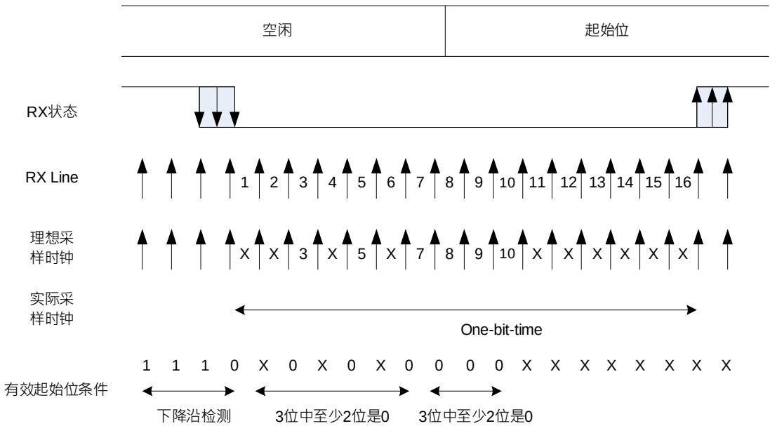
图 14-6 起始位侦测
