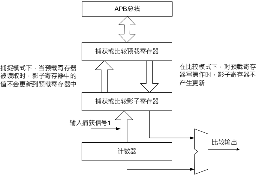
图 21-11 捕获或比较通道结构图
