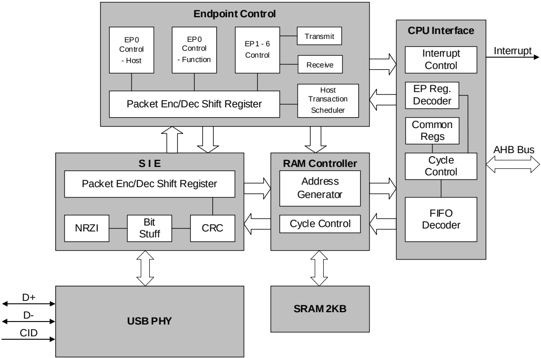
图 28-1 USB 结构图
