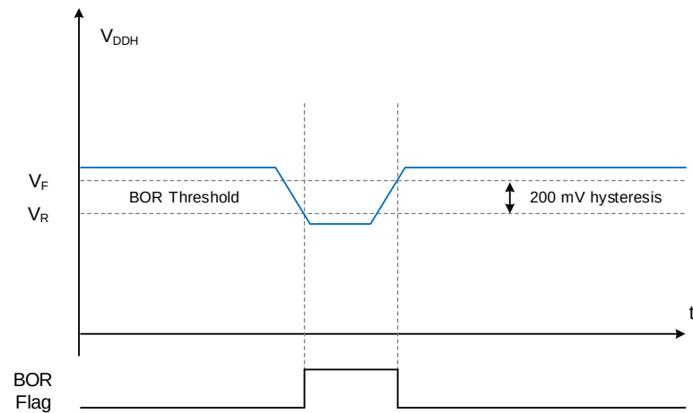
图 3-3 BOR 复位
