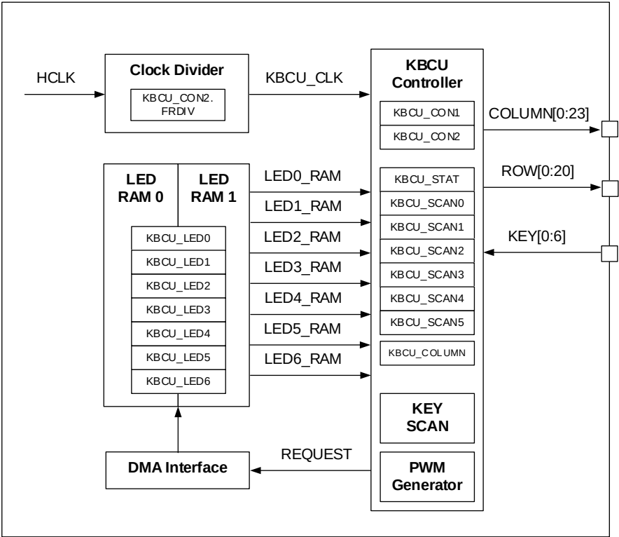
图 12-1 KBCU 结构图
