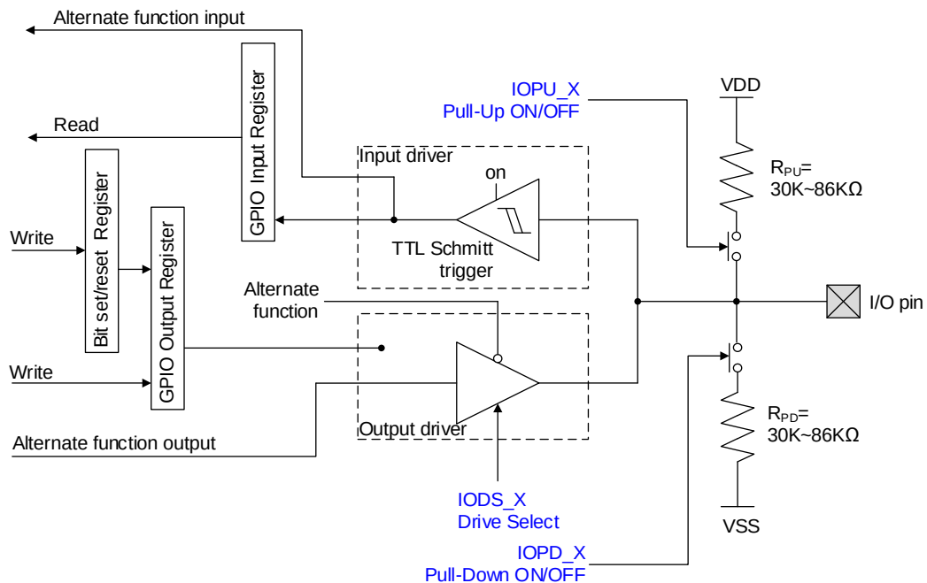
图 6-4 I/O 端口的复用配置
