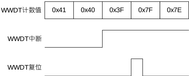
图 24-2 WWDT 中断示意图
