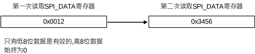
图 27-34 接收 0x123456
