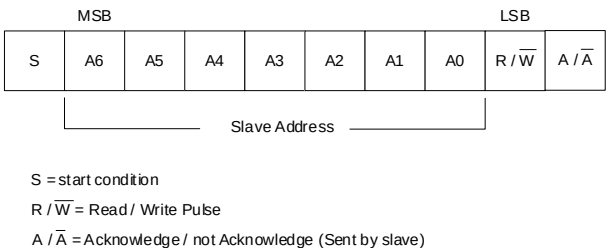
图 26-4 7 位地址格式
