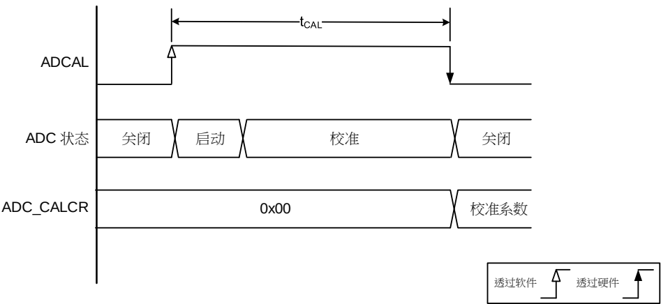
图 16-2 ADC 校准
