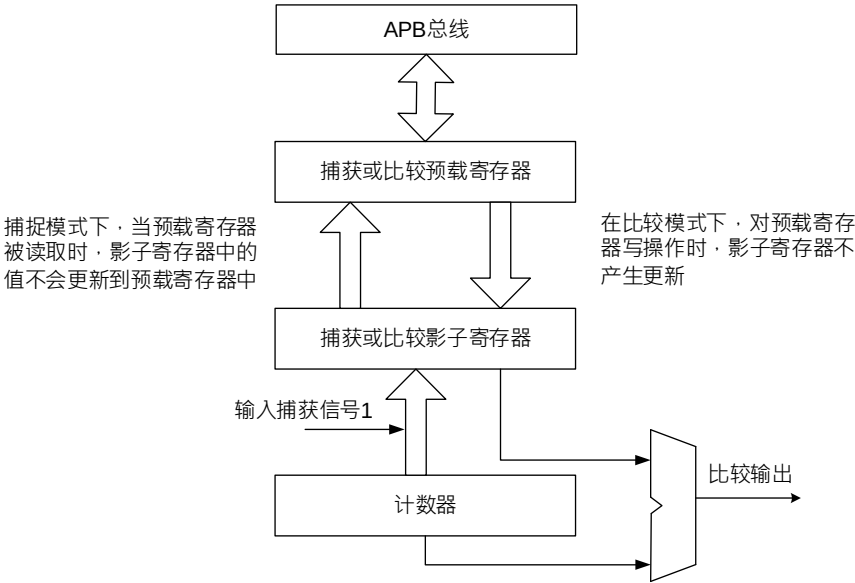
图 18-14 捕获或比较通道结构图
