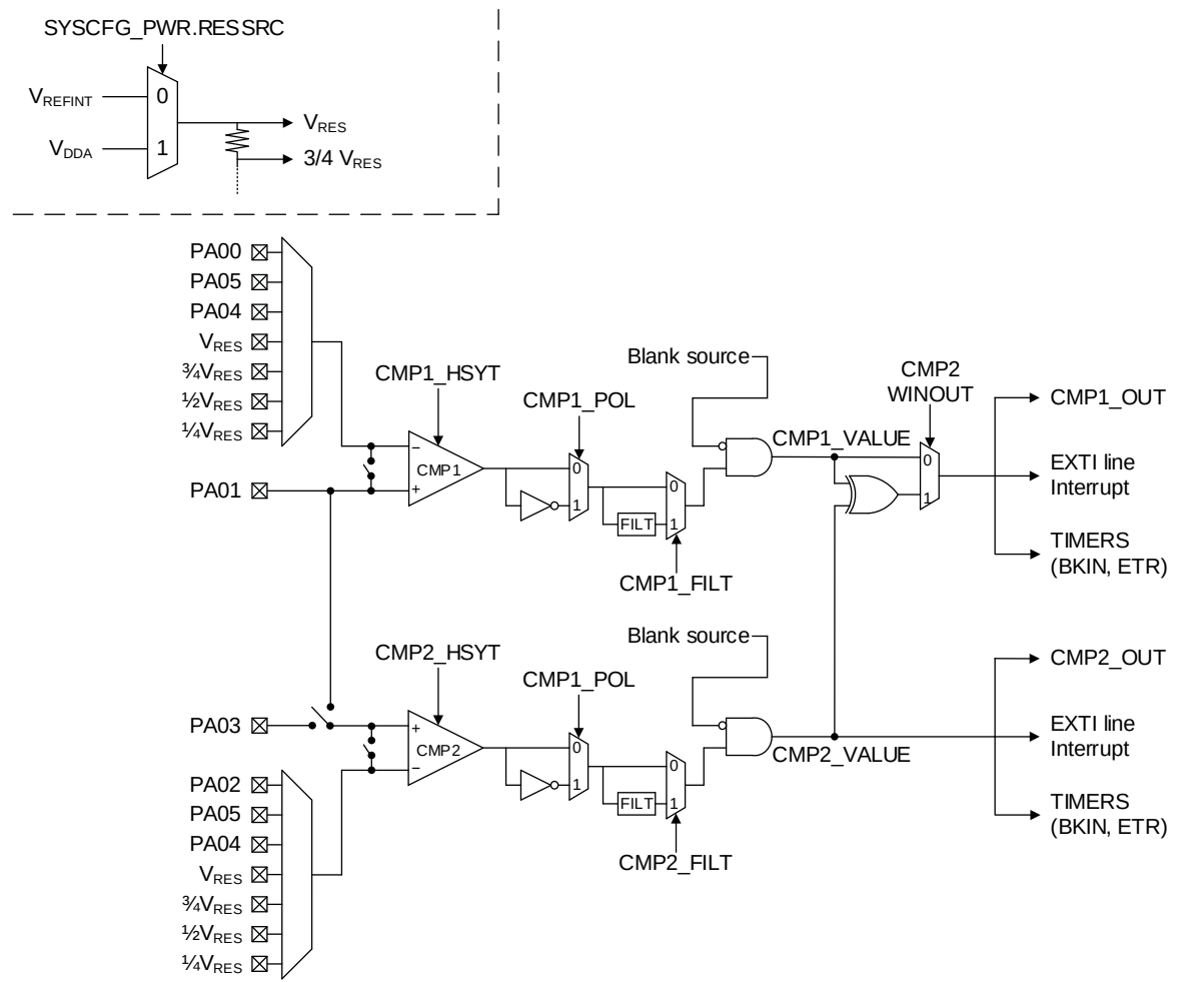
图 17-1 CMP 架构图
