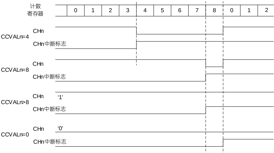
图 20-16 边沿对齐递增计数 PWM 波形（AR=8）
