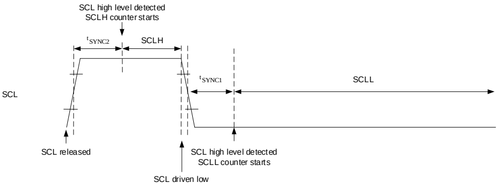
图 26-12 主机时钟产生
