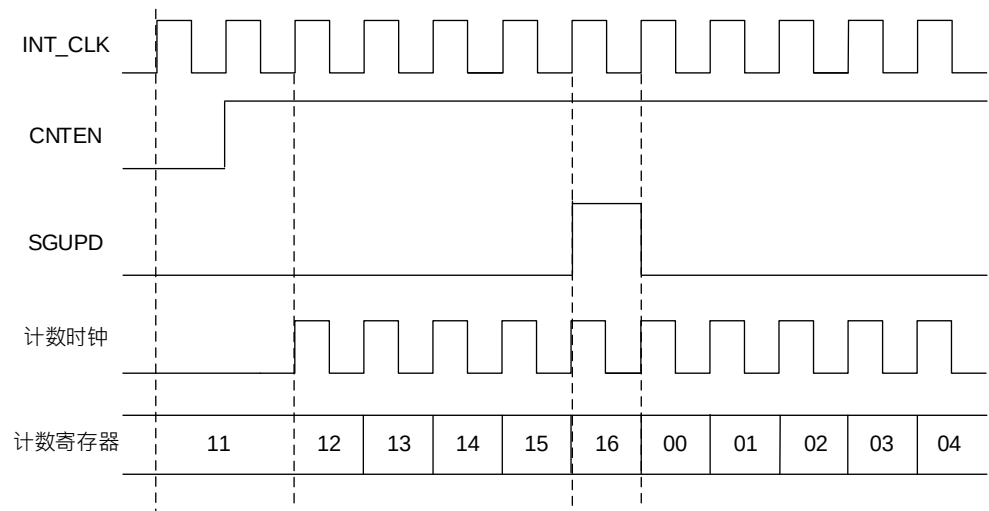
图 19-3 采用内部时钟计数
