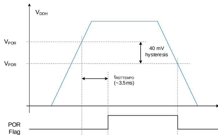
图 3-2 POR/PDR 复位
