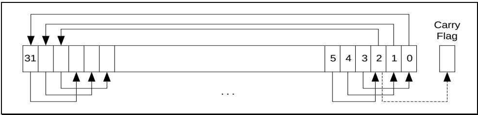
附录图 1-11ROR #3
