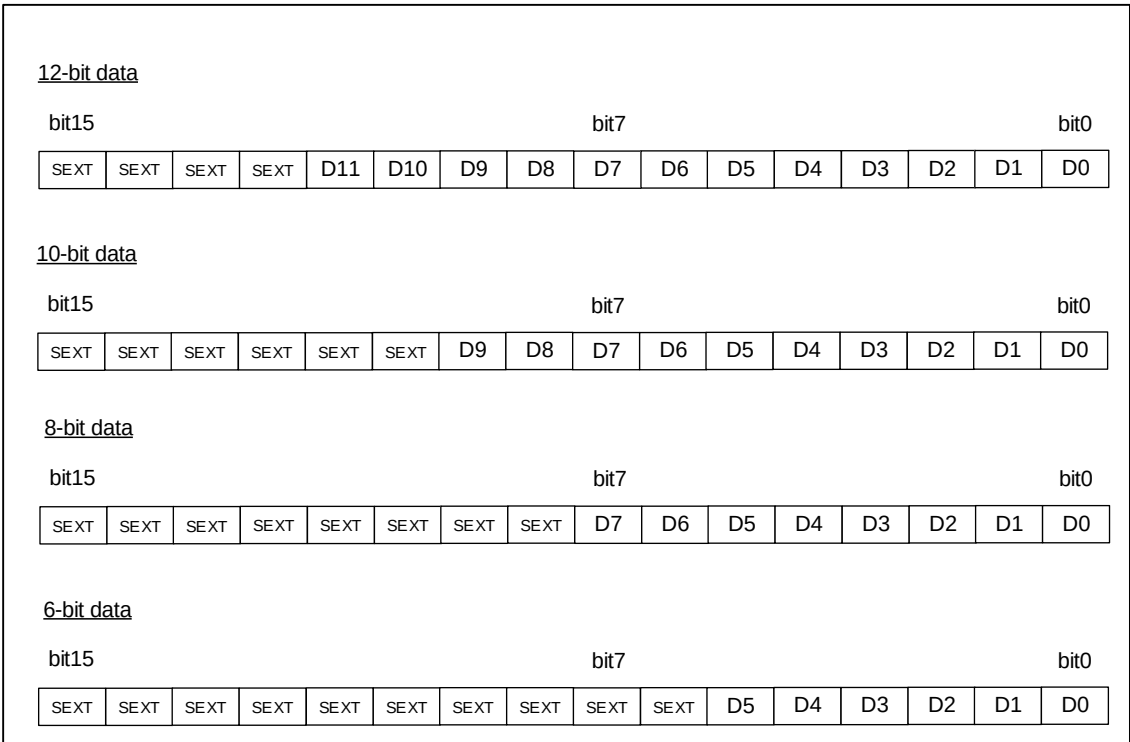
图 16-13 右对齐(使用偏移,有符号值)
