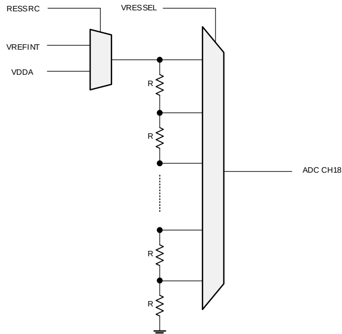
图 16-25 V_{RES} 分压
