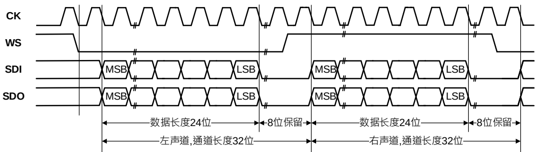
图 27-20 I2S 飞利浦标准波形(24 位数据帧，CKPOL = 0)
