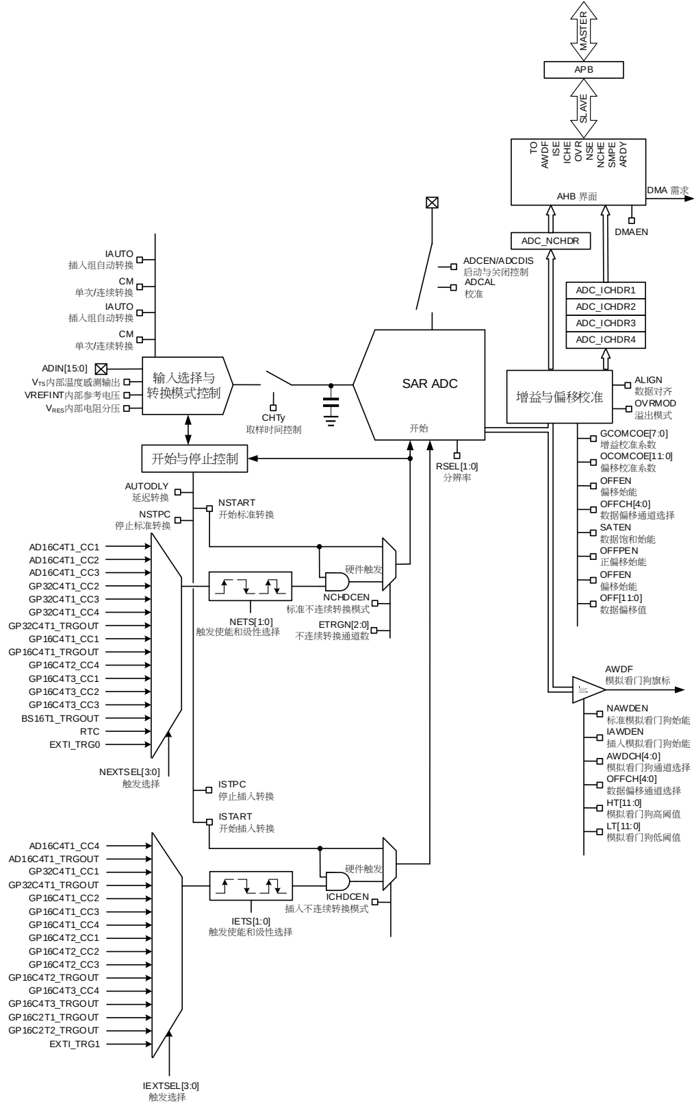
图 16-1 ADC 结构图
