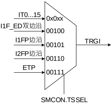
图 19-6 ITn 内部时钟连接
