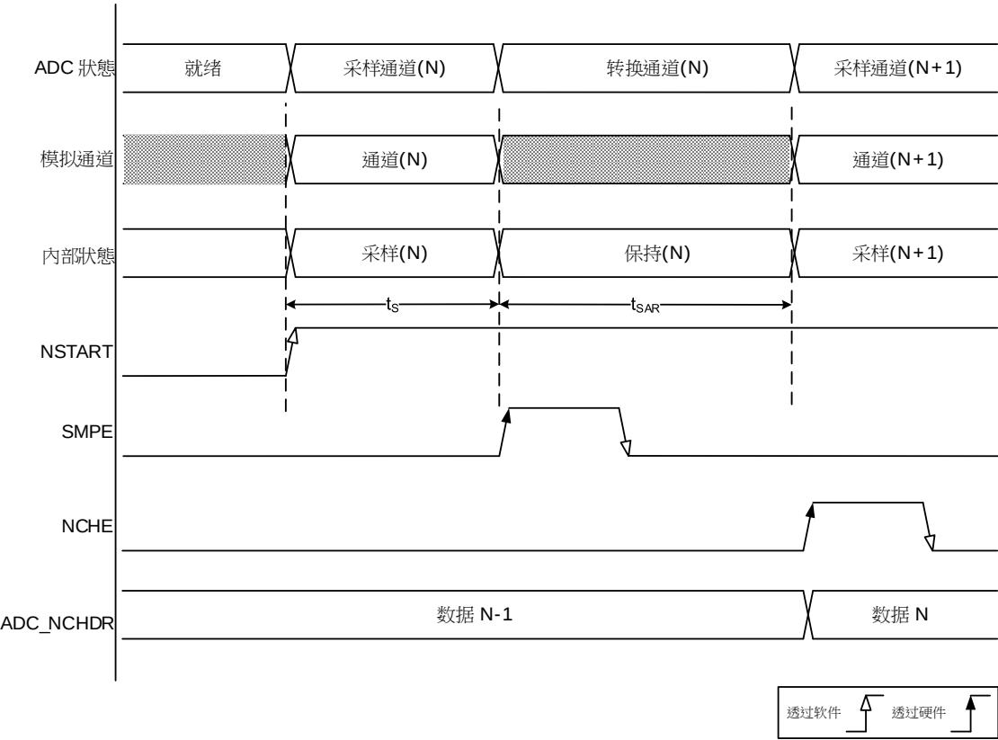
图 16-4ADC 标准转换
