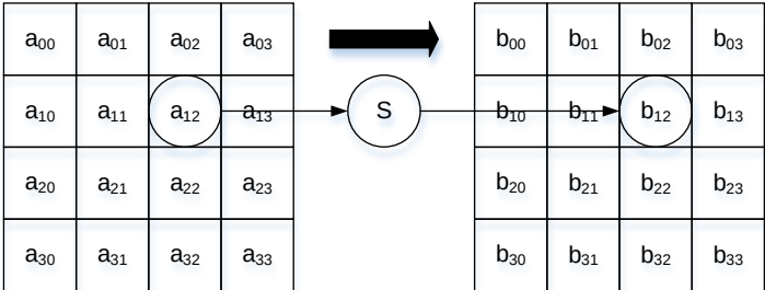
图 9-2 字节代换
