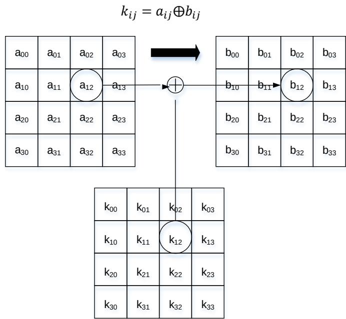
图 9-1 轮密钥加
