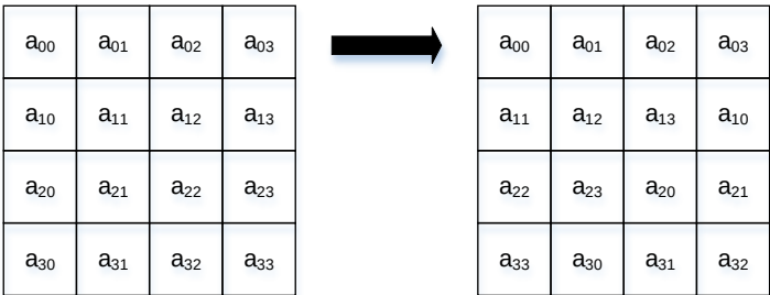
图 9-3 行移位
