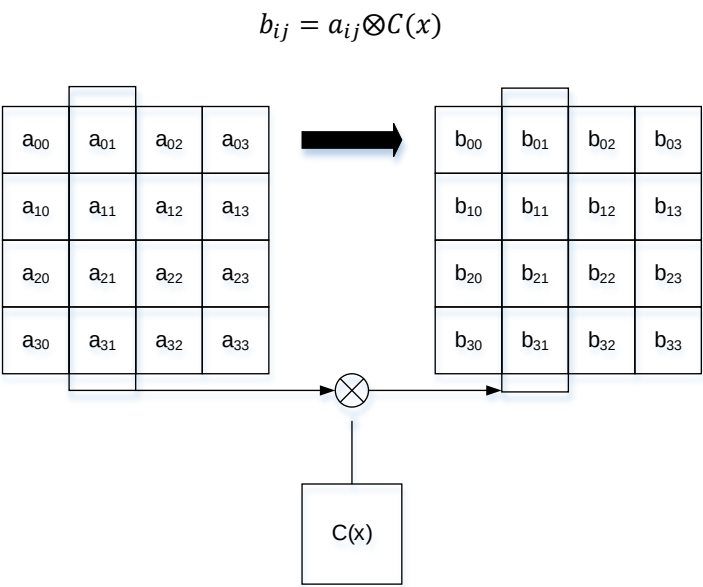
图 9-4 列混合
