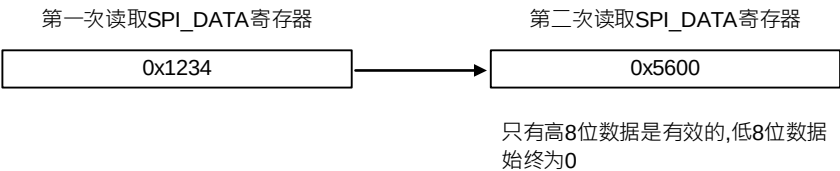
图 27-28 接收 0x123456
