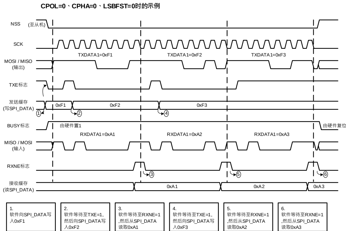
图 27-8 全双工通信(SPI_CON1.BIDEN=0 且 SPI_CON1.RXO=0)的 TXE、RXNE、BUSY 行为(直接存取操作模式在连续传输的情况下)
