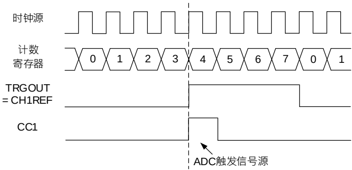
图 18-37ADC 触发生成
