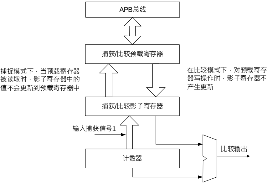
图 19-13 捕获或比较通道结构图
