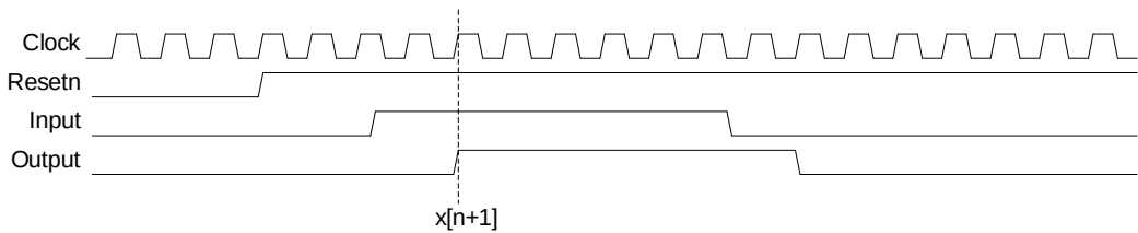
图 14-5 防抖动输出
