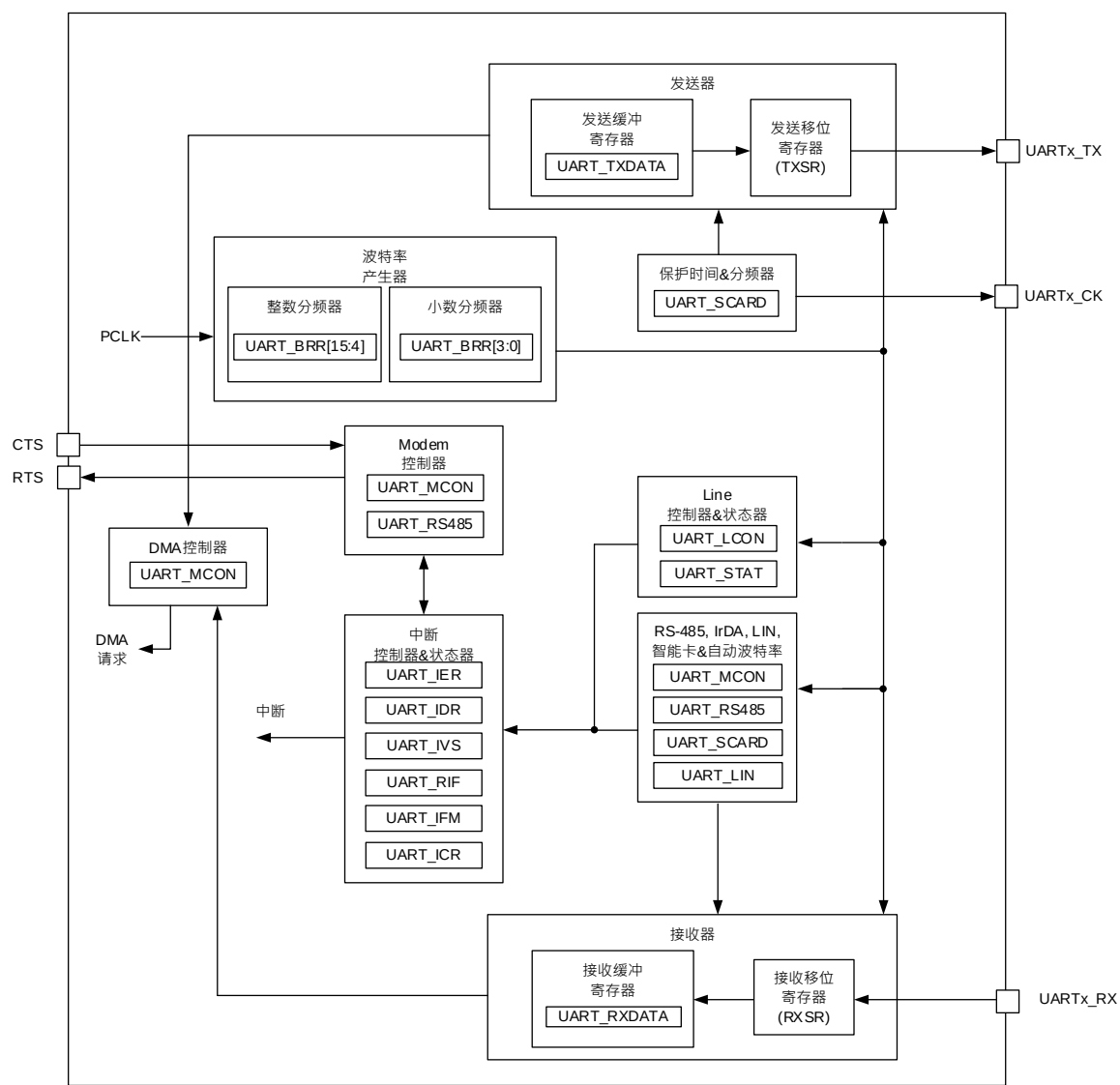
图 14-1 UART 框图
