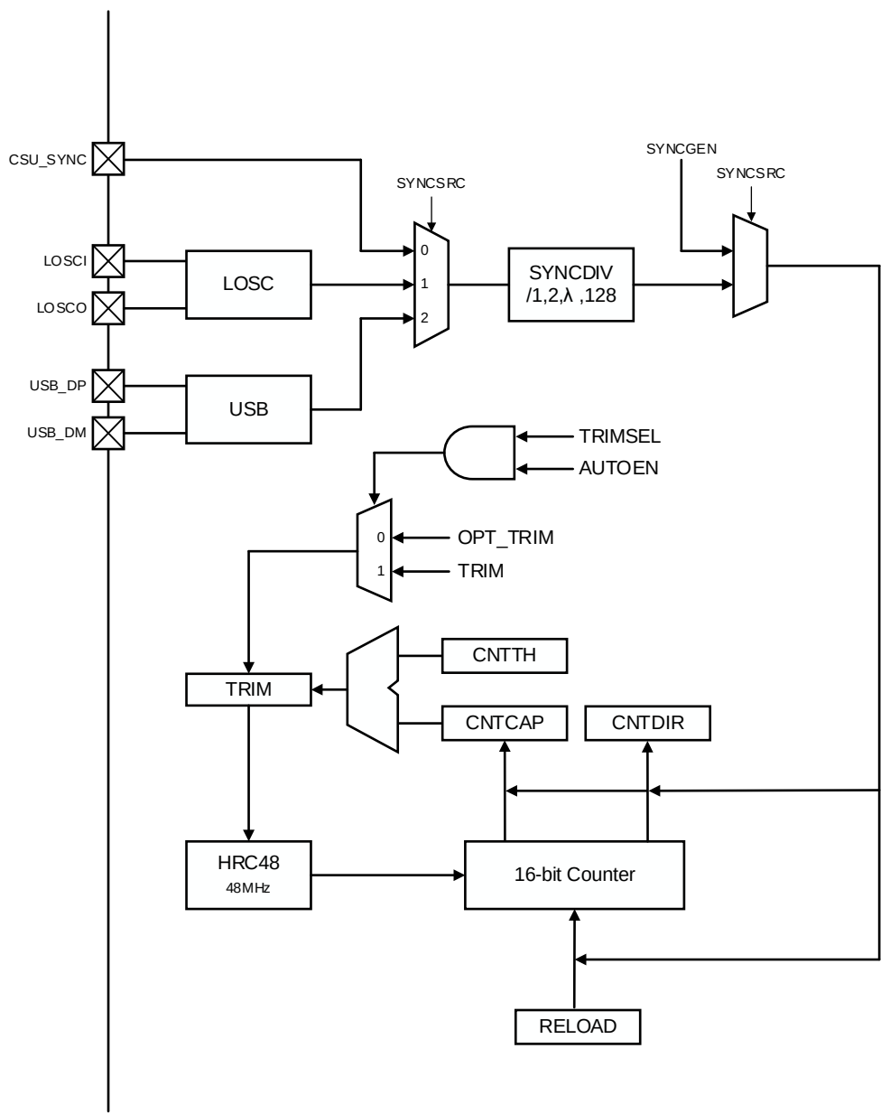
图 11-1 CSU 结构图
