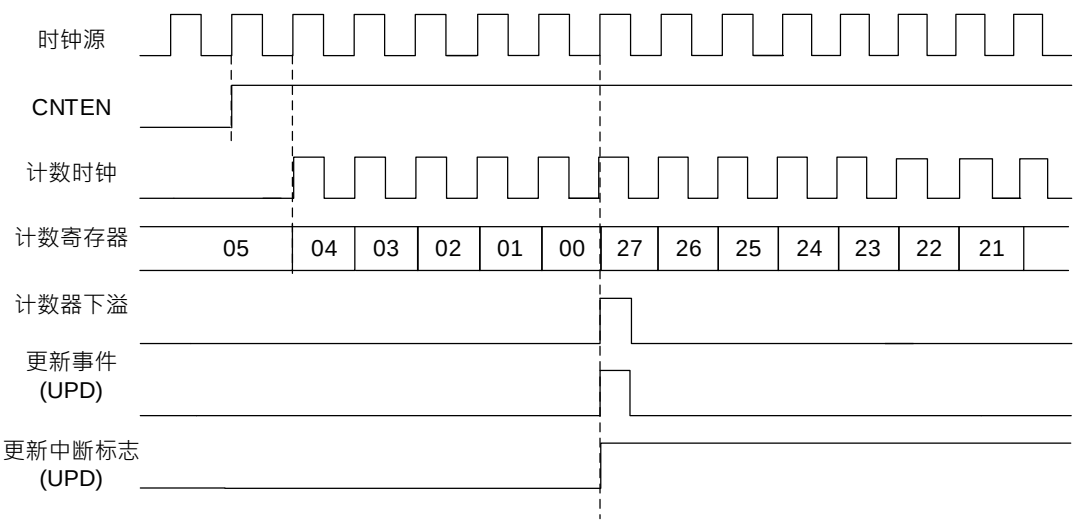
图 20-10 计数器递减计数时序图
