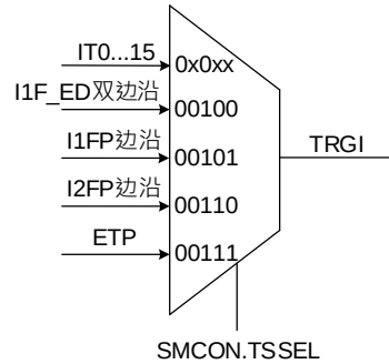
图 20-6 ITn 内部时钟连接
