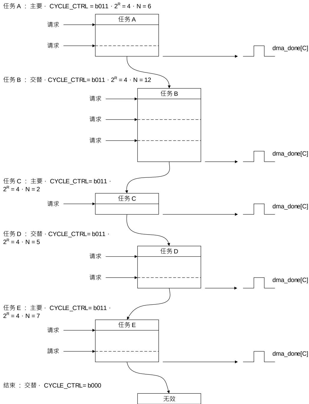
图 13-3 乒乓示例图
