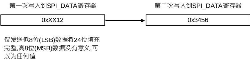
图 27-33 发送 0x123456
