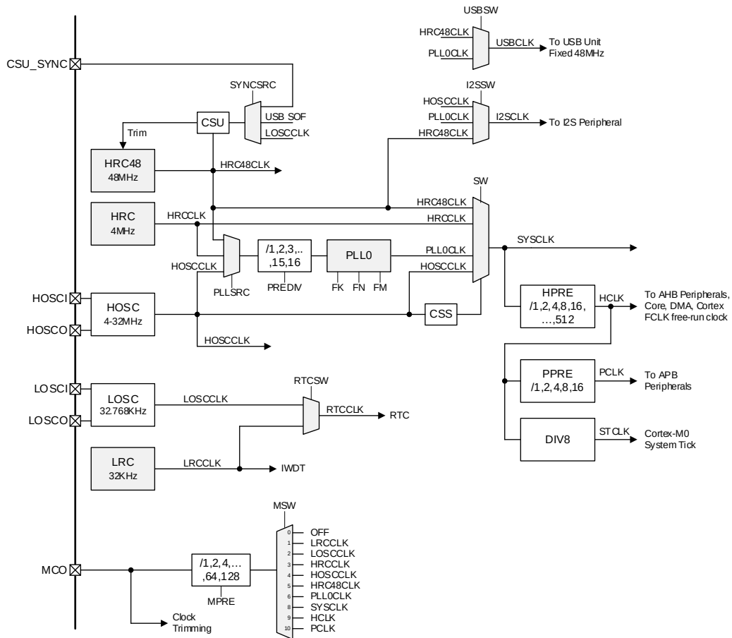
图 4-2 时钟架构图
