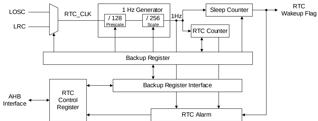
图 25-1 RTC 架构图
