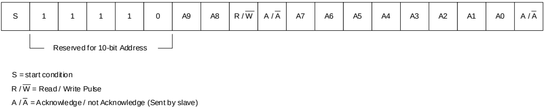
图 26-5 10 位地址格式
