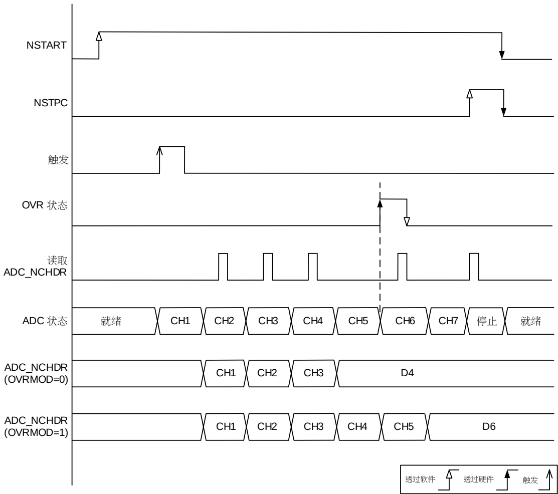
图 16-16 溢出示意图
