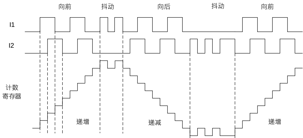
图 20-22 编码器接口模式下的计数操作
