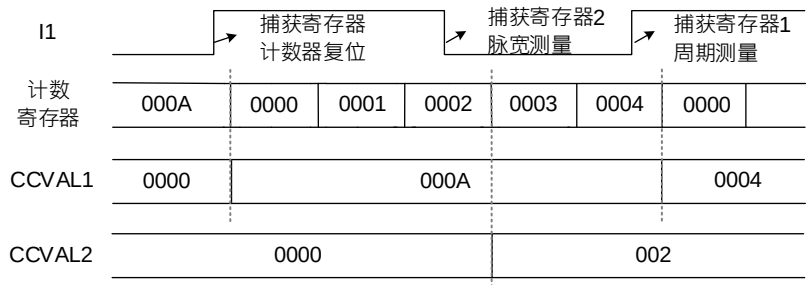
图 21-13 PWM 输入模式时序
