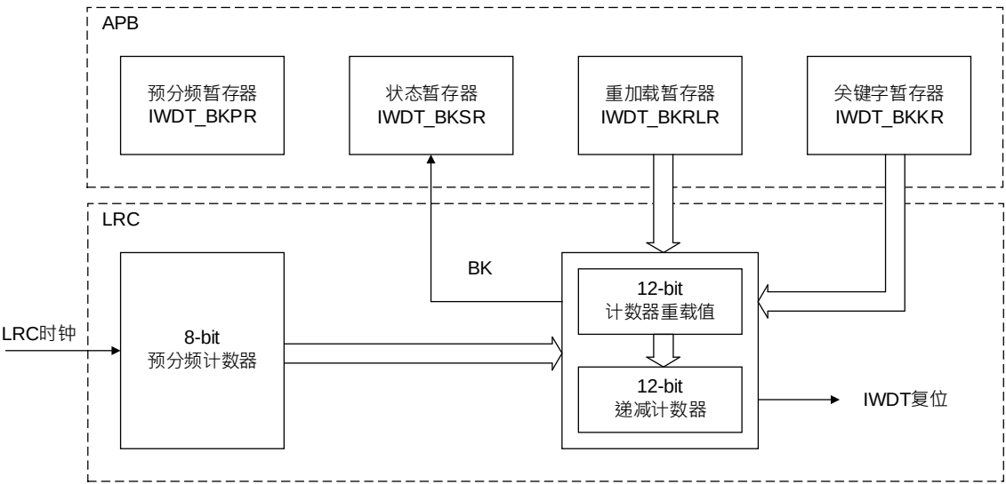
图 23-1IWDWT 架构图
