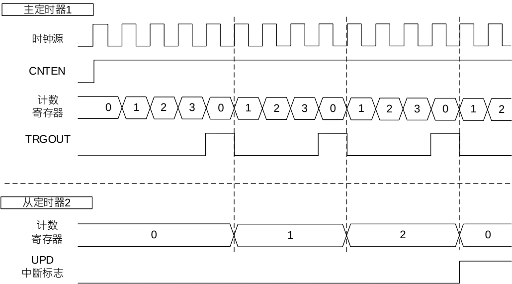
图 21-25 使用主定时器更新事件触发从定时器计数
