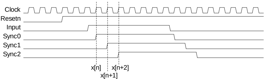
图 14-4 防抖动波形
