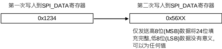
图 27-21 发送 0x123456
