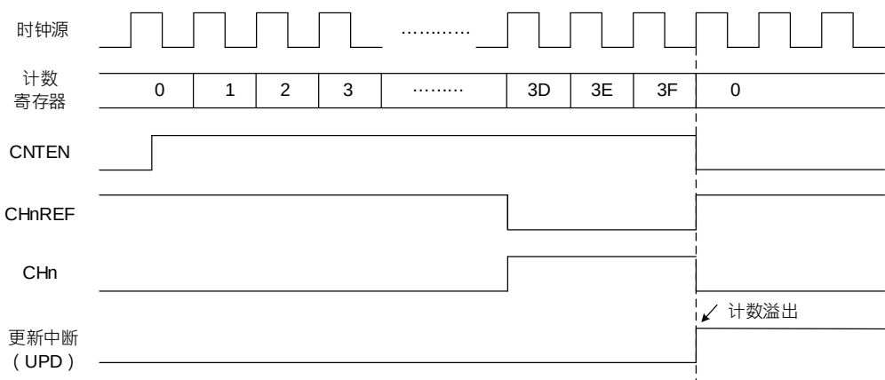
图 18-22 单脉冲模式
