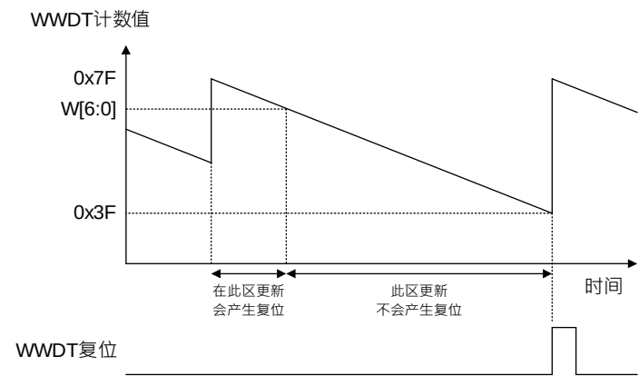
图 24-3WWDT 时序图
