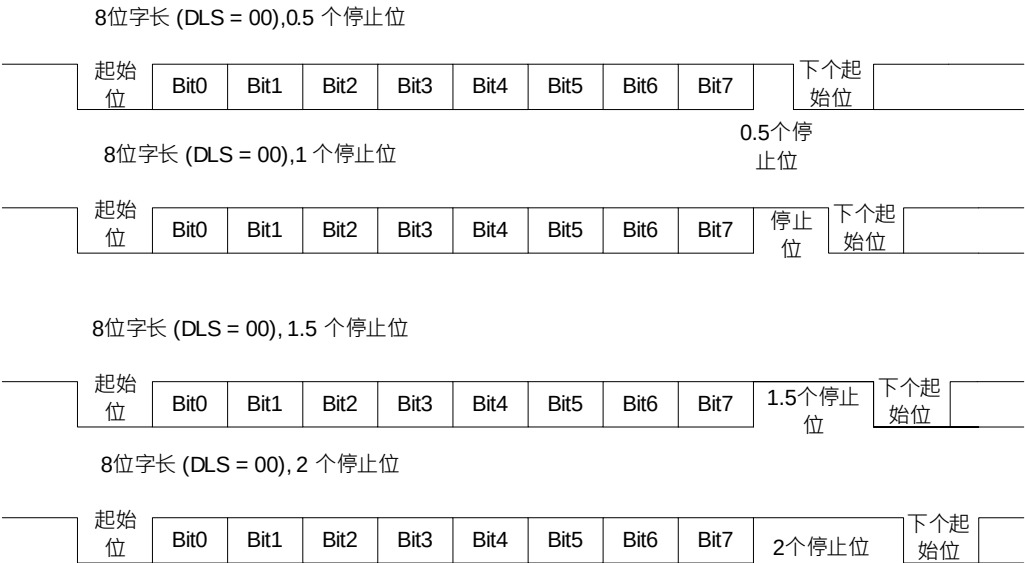
图 14-3 配置停止位
