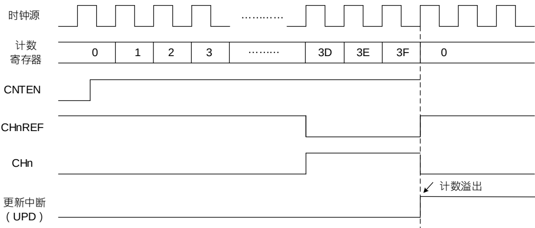
图 21-16 单脉冲模式
