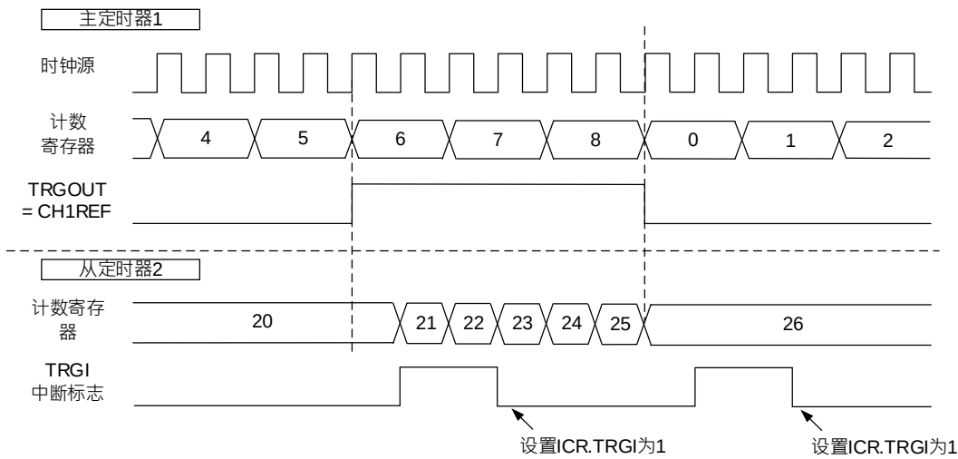
图 19-29 门控从定时器使用主定时器 CH1REF
