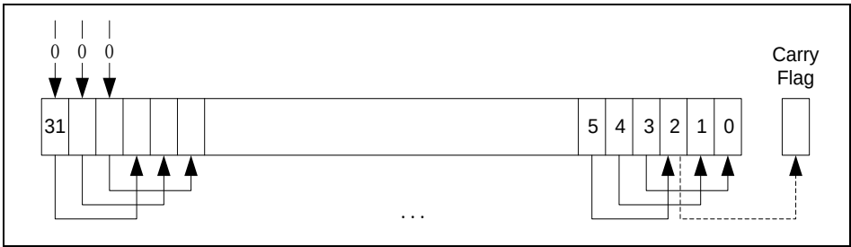
附录图 1-9LSR #3
