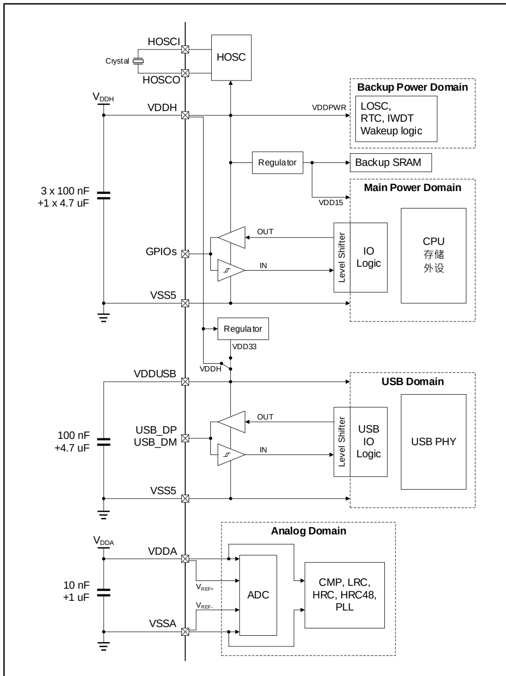
图 3-1 电源架构
