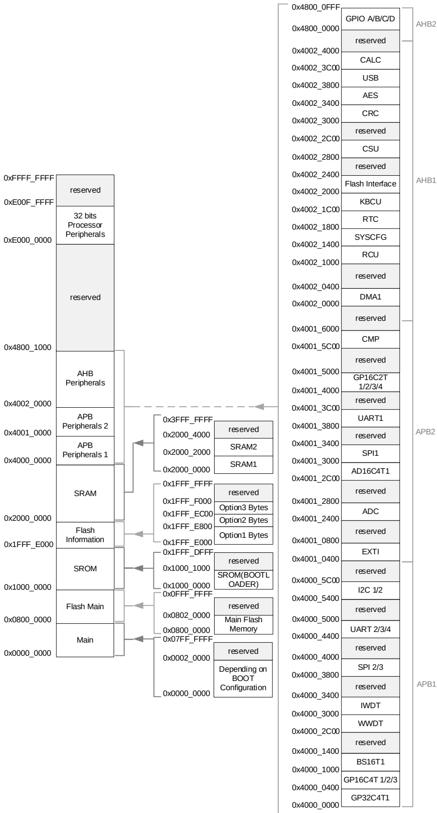
图 1-2 内存映射
