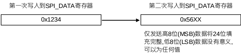
图 27-27 发送 0x123456
