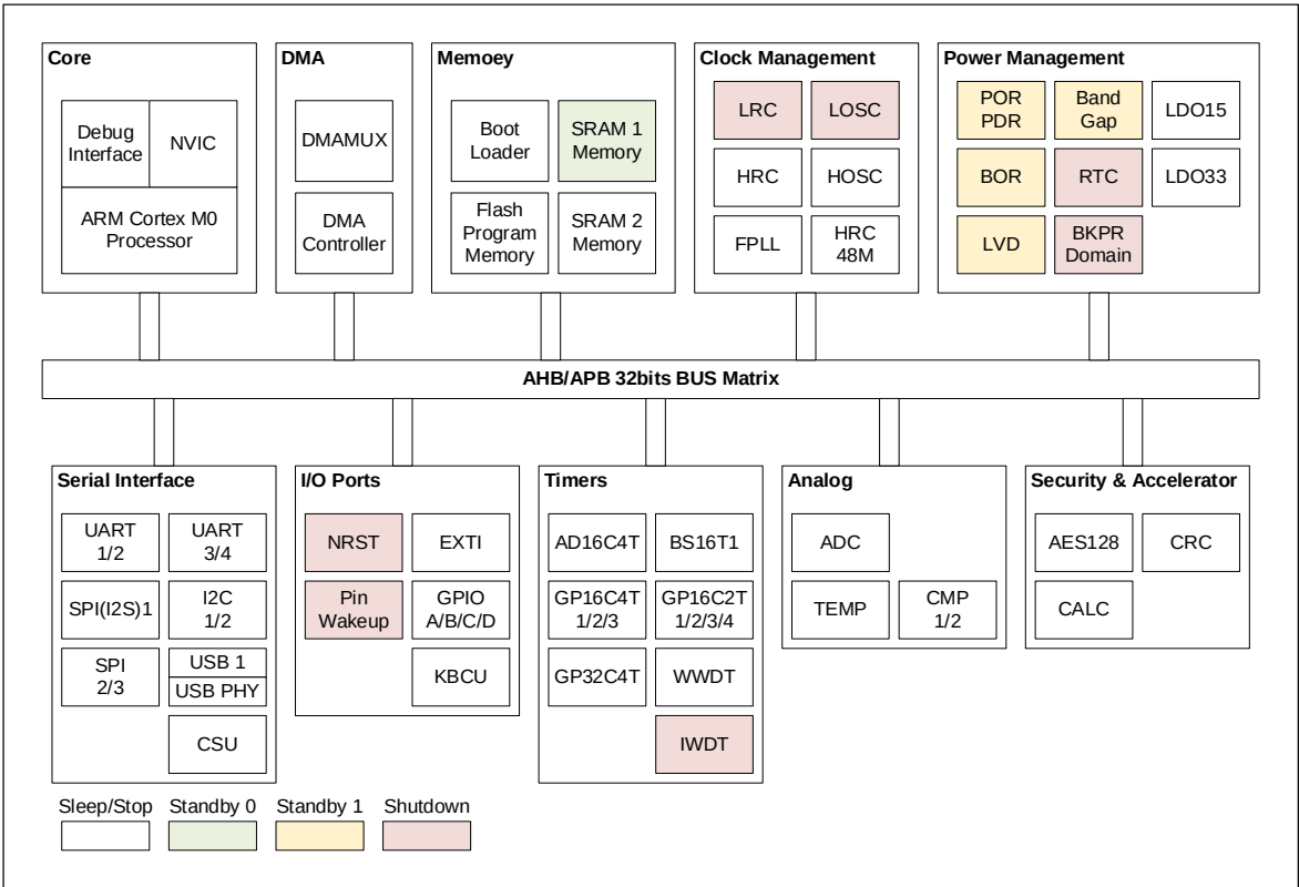
图 1-1FS026x7L 系统框图
