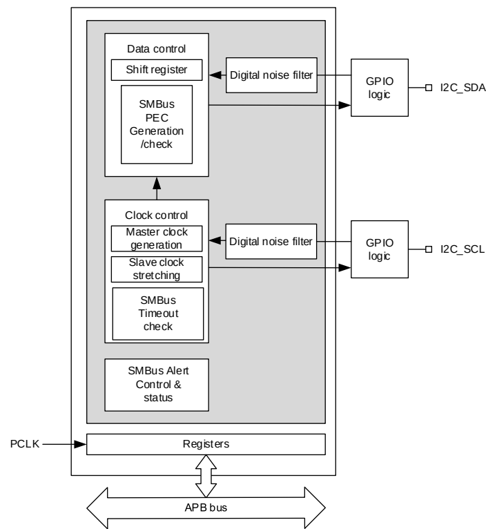
图 26-1 I2C 结构图
