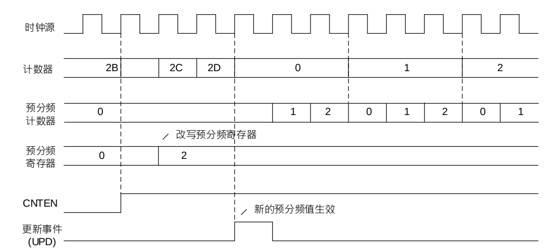
图 19-2 预分频值计数时序图
