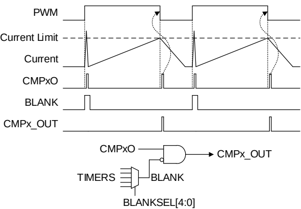
图 17-4 消隐功能示意图
