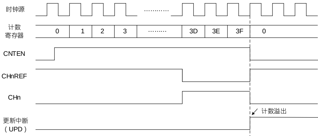
图 20-21 单脉冲模式
