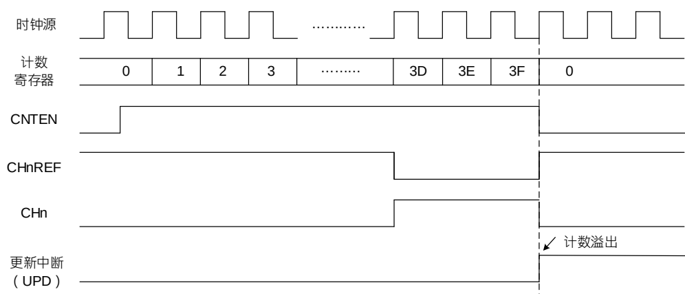
图 19-21 单脉冲模式
