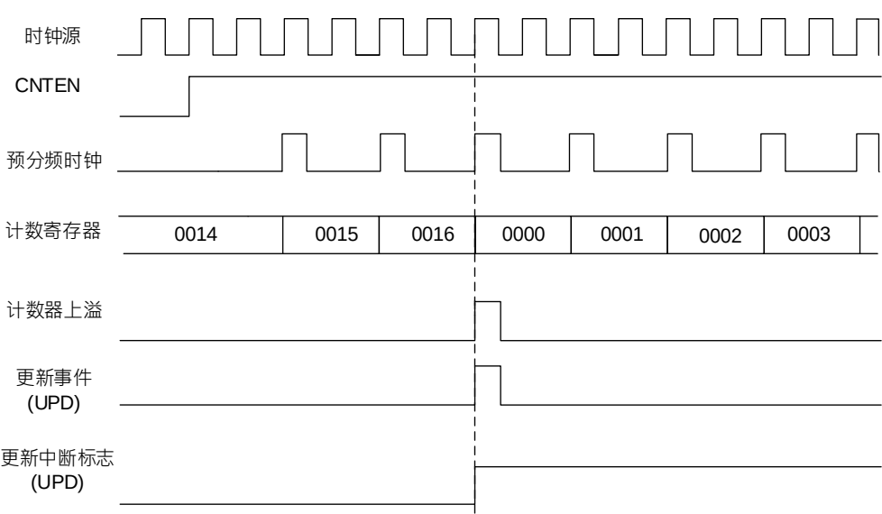
图 22-4 计数器递增计数时序图
