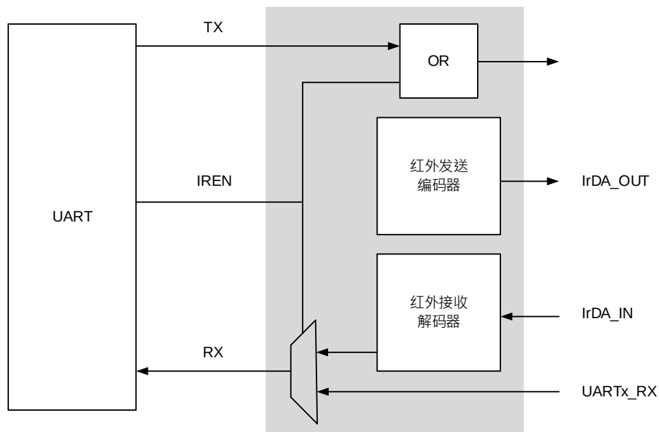
图 14-20 红外收发框图
