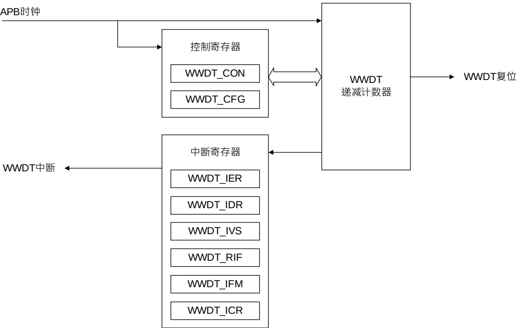
图 24-1WWDT 架构图
