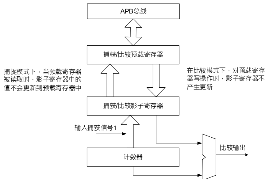
图 20-13 捕获或比较通道结构图
