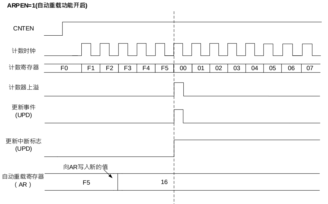
图 18-10 设置 ARPEN 位为 1 时计数器时序图
