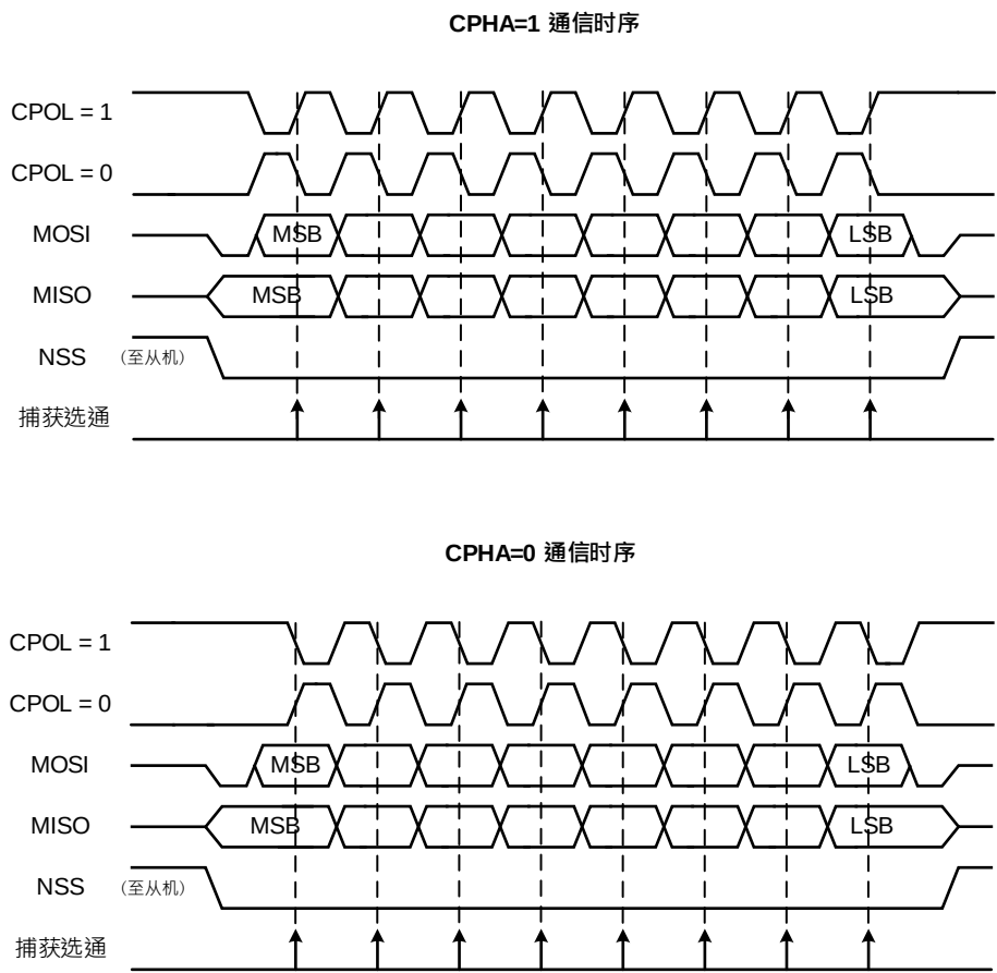
图 27-2 SPI 格式
