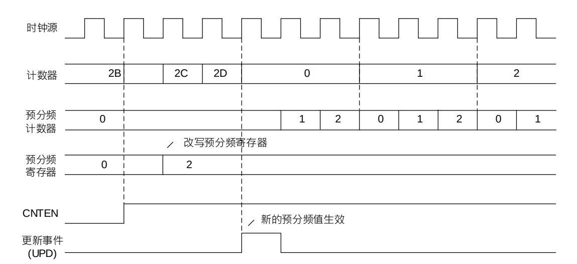
图 22-2 预分频值计数时序图
