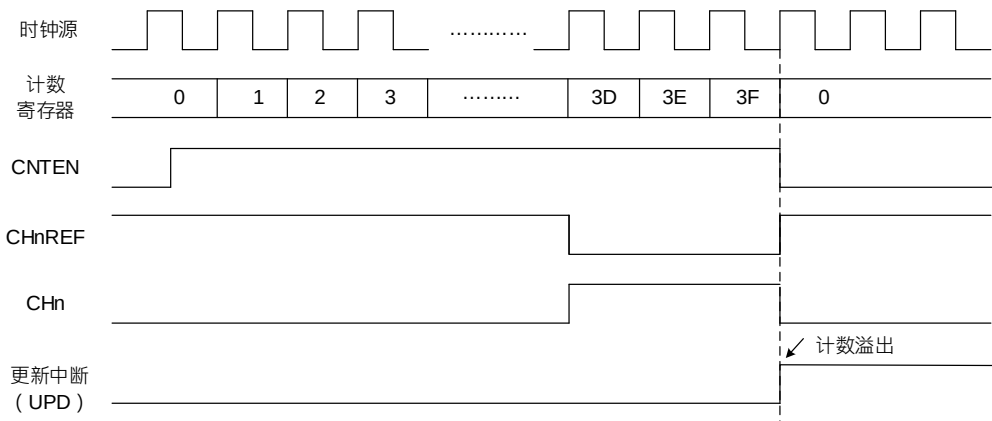
图 19-21 单脉冲模式
