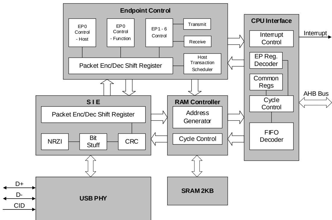
图 28-1 USB 结构图
