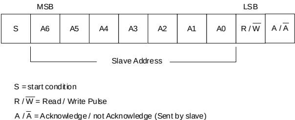
图 26-4 7 位地址格式
