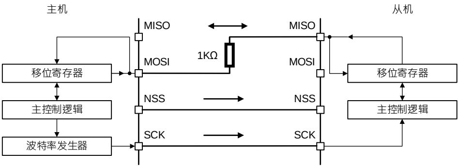
图 27-4 半双工通信
