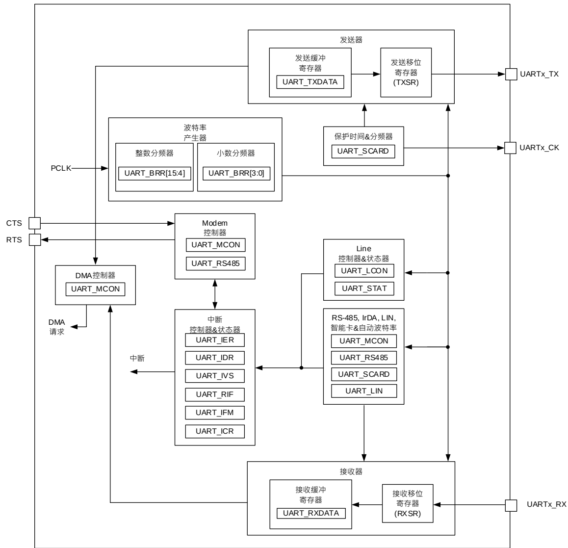
图 14-1 UART 框图
