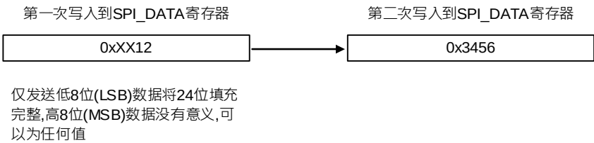
图 27-33 发送 0x123456
