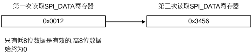
图 27-34 接收 0x123456
