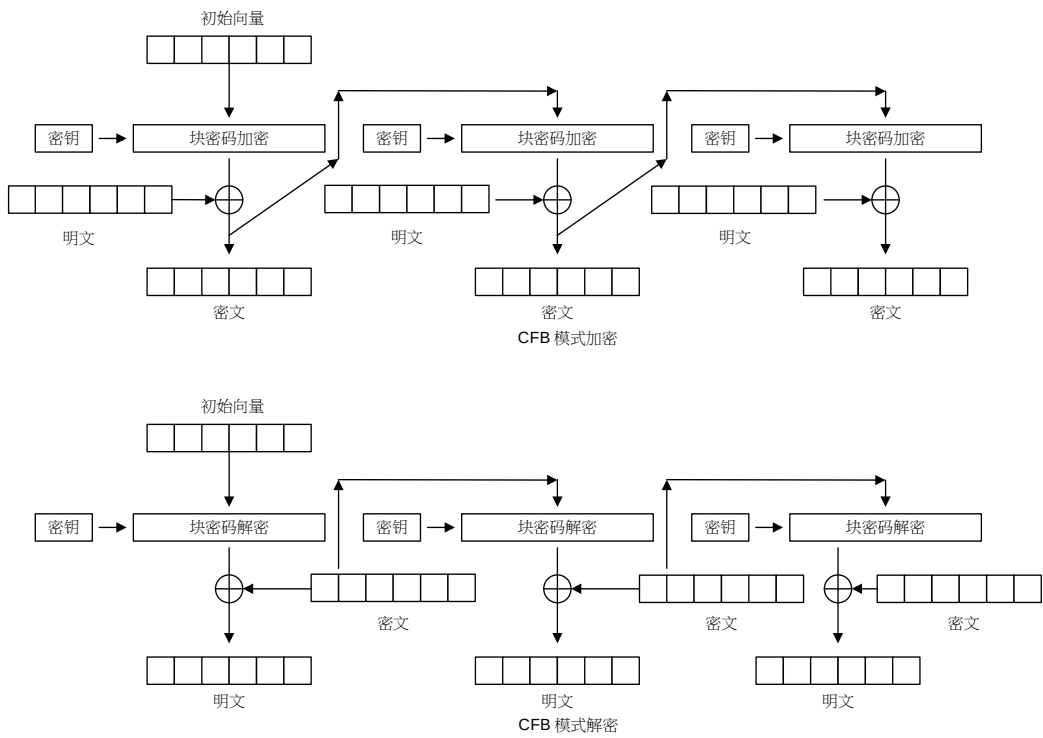
图 9-10 CFB 模式
