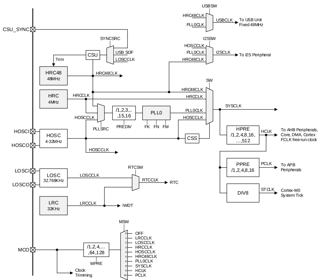
图 4-2 时钟架构图
